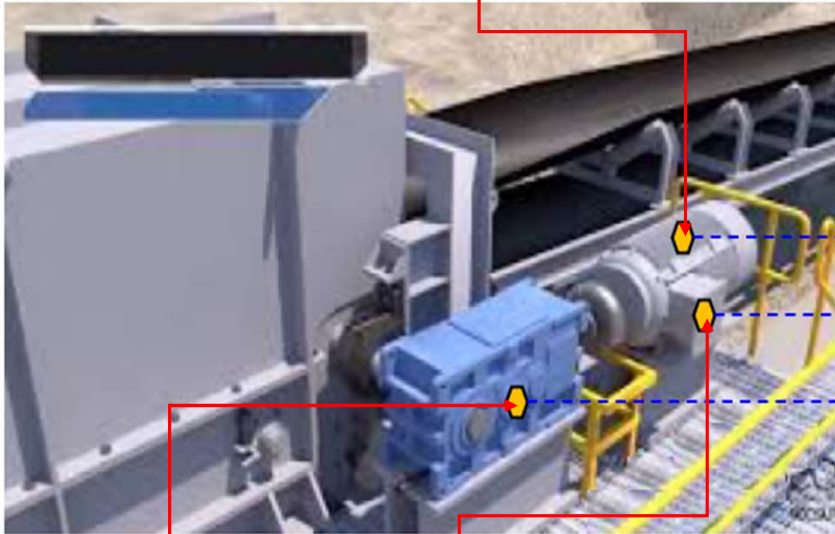
Sensor de temperatura en reductor 2 de faja tubular
